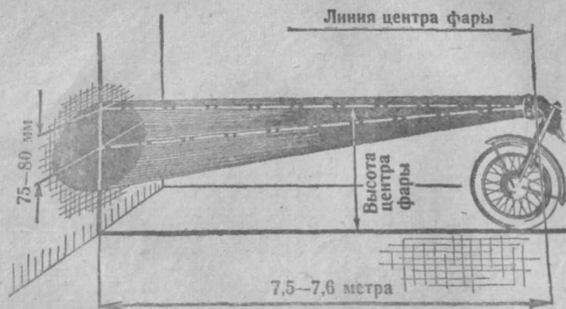
Рис. 37. Регулировка фары
