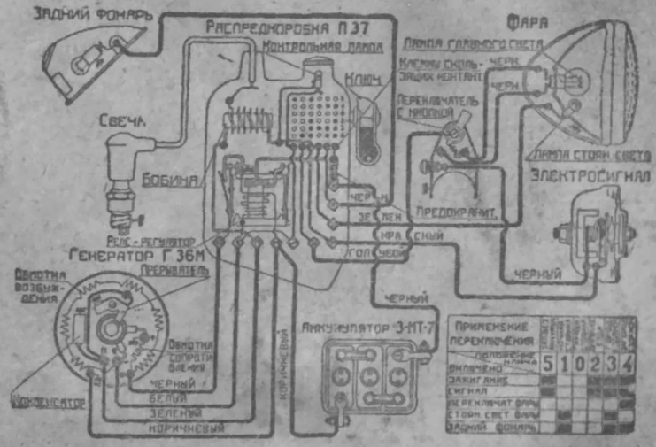
Рис. 26 Схема электрооборудования
